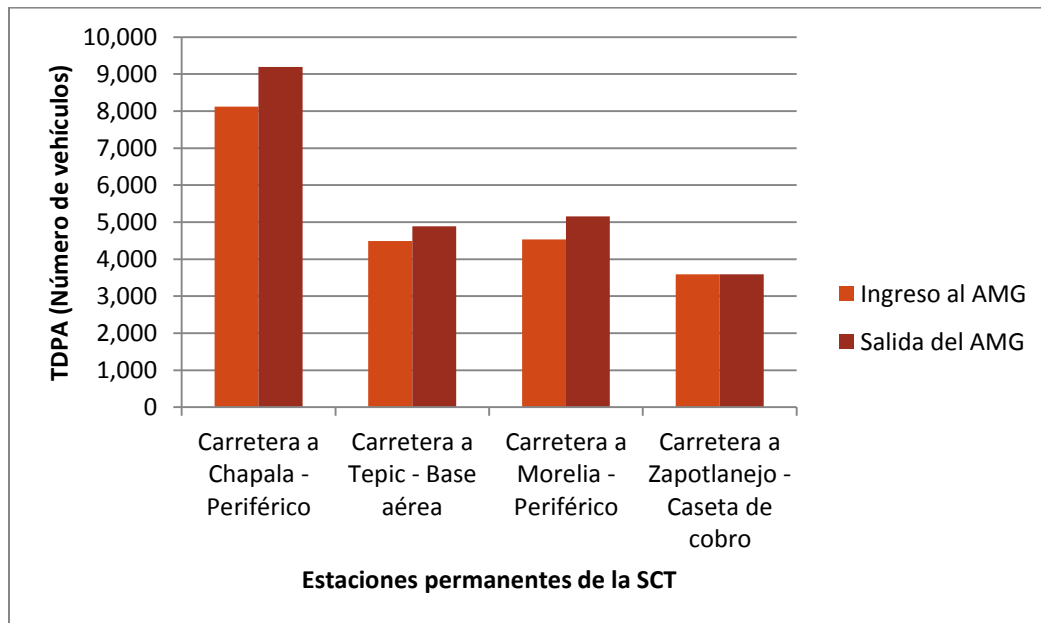
Gráfica 18.-TDPA de vehículos de carga que circulan en los principales accesos carreteros de acuerdo a estaciones permanentes de SCT.
