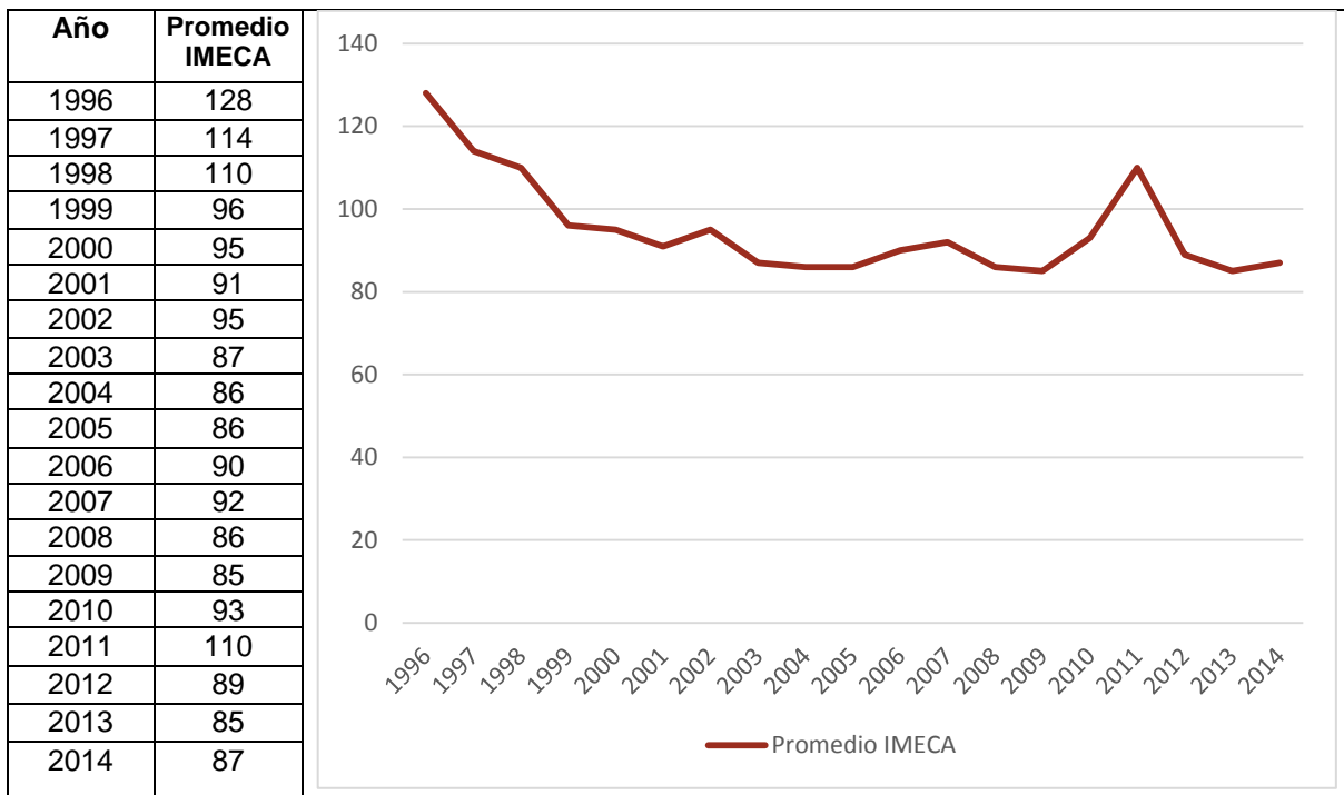
Gráfica 19.-Promedio de IMECAS 1996-2014 en el AMG.
