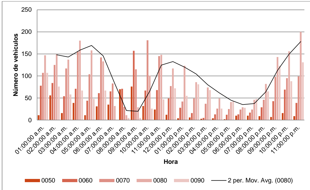
Gráfica 8.-Espectro de las velocidades a las que circulan los vehículos a lo largo del día sobre el Anillo Periférico, 2014.
